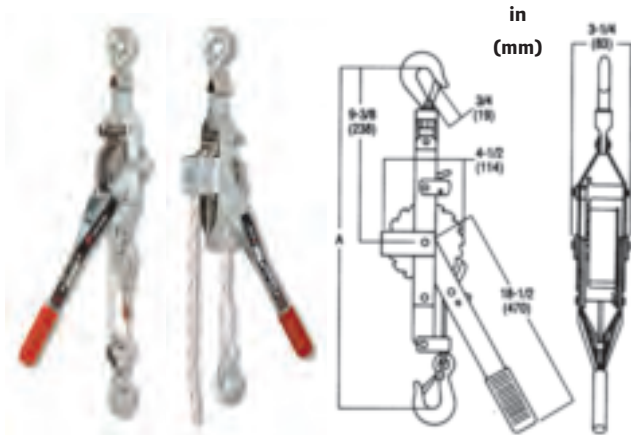
P-Series Pullers
